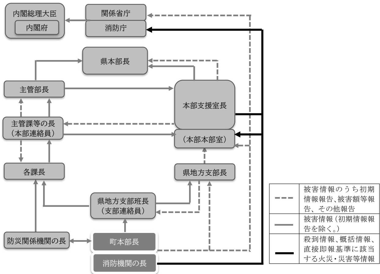
資料編3-4-2 報告区分別系統図
